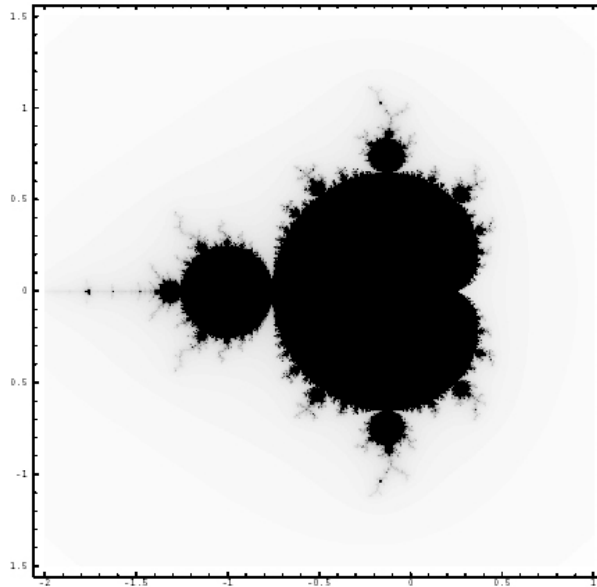
Рисунок 11. Построение Мандельброта
