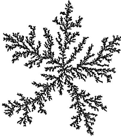
Рисунок 15. Фрактальный кластер
