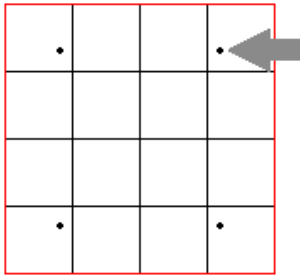
Рисунок 35. Аттракторы Грязнуши
