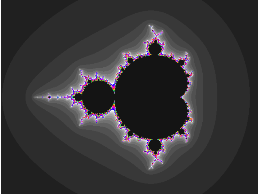
Рисунок 6. Построение Мандельброта
