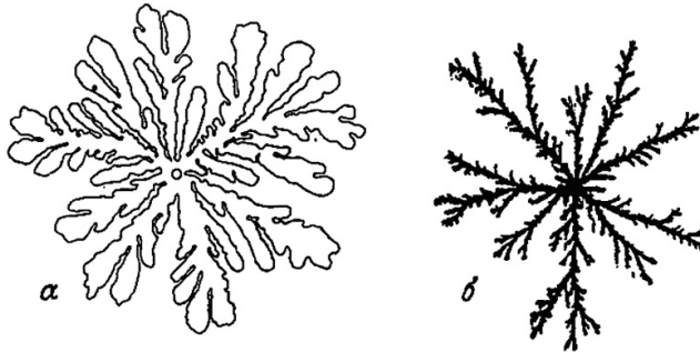
Рисунок 14. Вязкие пальцы
