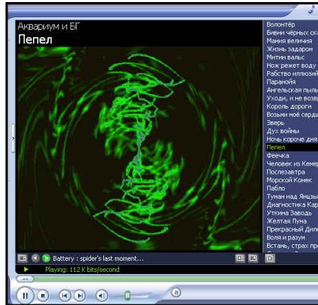
Рисунок 5. «Цветомузыка»
