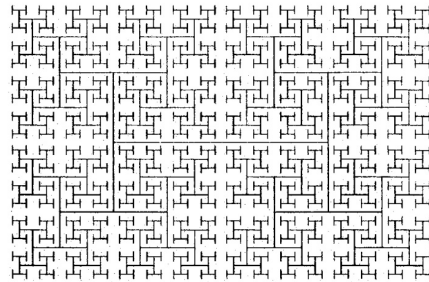
Рисунок 4. Н-фрактал
