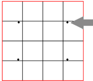
Рисунок 36. Аттракторы Семёновки
