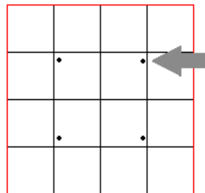
Рисунок 36. Аттракторы Семёновки
