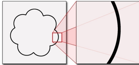
Рисунок 2. Немасштабируемая фигура
