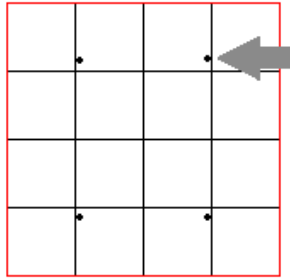
Рисунок 34. Аттракторы Сосновки
